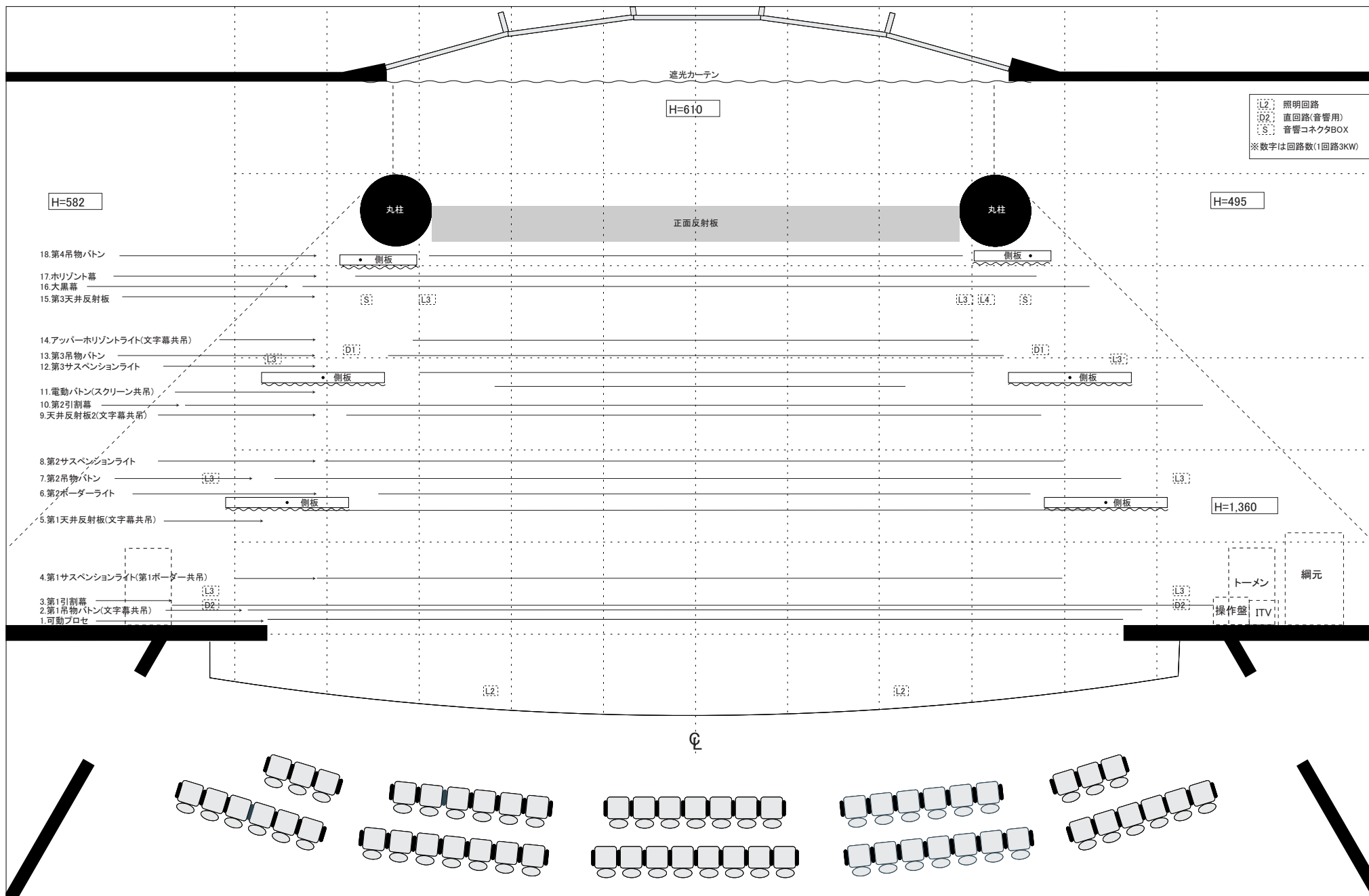
図面2 舞台平面図(1間単位)
